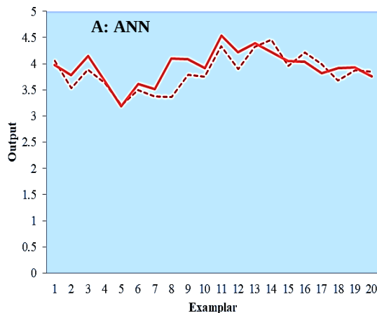
شکل ۶. نتایج تست شبکه‌های عصبی مصنوعی برای تخمین سطوح ریسک (محورهای افقی و عمودی بیانگر مقادیر ریسک واقعی و پیش‌بینی شده به صورت نرمال شده در بازه [۰،۱] و بدون بُعد می‌باشند).
