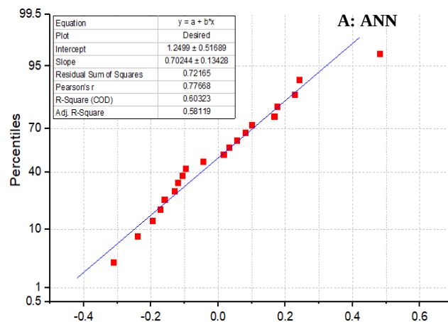
شکل ۷. نتایج باقیمانده‌های نرمال برای شبکه‌های مطلوب ANN (A) و RBF (B)
