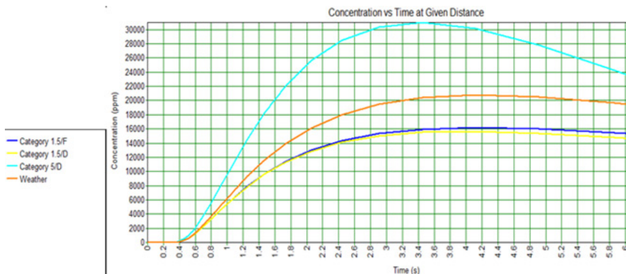
شکل ۲. نمودار میزان غلظت گاز متان (پی پی ام) برحسب زمان در فاصله ۱۰ متری از مخازن در صورت ایجاد ترکیدگی فاجعه بار مخزن
