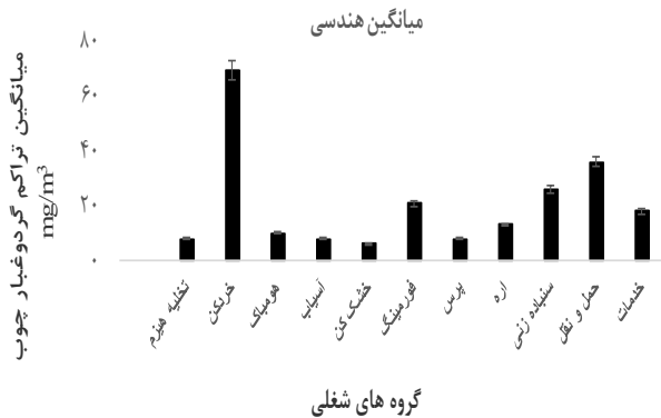
نمودار ۱. میزان مواجهه گروه های شغلی مختلف با گردوغبار استنشاقی (میلی گرم بر مترمکعب)
