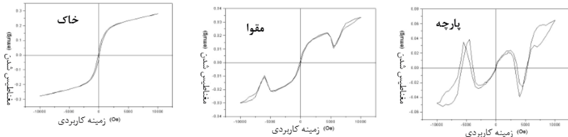
شکل ۲) نمودار حلقه های پسماند مغناطیسی نمونه های خاک، مقوا و پارچه
