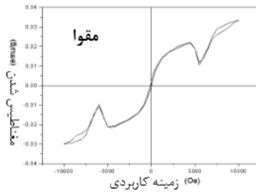
شکل ۲) نمودار حلقه های پسماند مغناطیسی نمونه های خاک، مقوا و پارچه
