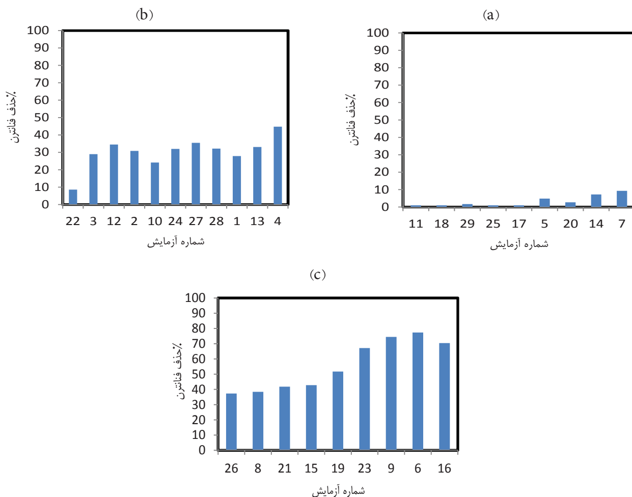
شکل ۲- میزان حذف در آزمایشات مختلف (a) غلظت سورفاکتانت ۵۰۰ mg/l (b) غلظت سورفاکتانت ۲۷۵۰ mg/l (c) غلظت سورفاکتانت ۵۰۰۰ mg/l در آزمایشات ۱۱، ۱۸، ۲۹، ۲۵، ۲۶، ۸، ۲۱، ۱۵. L/S= ۲۰ ml/g در آزمایشات ۱۷، ۳، ۱۲، ۲، ۱۰، ۲۴، ۲۷، ۲۸، ۱، ۱۳، ۱۹. L/S= ۱۰ ml/g در آزمایشات ۵، ۲۰، ۱۴، ۷، ۴، ۲۳، ۱۶. در آزمایشات ۱۱، ۱۸، ۲۹، ۵، ۱۴، ۱۲، ۲۶، ۲۱، ۲۳، ۶. HA= ۱۰ mg/l در آزمایشات ۱۷، ۳، ۲، ۱۰، ۲۴، ۲۷، ۲۸، ۱۳، ۴، ۱۹. HA= ۲۰ mg/l در آزمایشات ۱۸، ۲۵، ۲۰، ۷، ۱، ۸، ۱۵، ۱۶. زمان شستشو= ۲ h در آزمایشات ۱۱، ۱۸، ۵، ۲۰، ۳، ۲۶، ۸، ۲۳، ۹. زمان شستشو= ۱۳ h در آزمایشات ۱۷، ۳، ۲، ۱۲، ۲، ۱۰، ۲۴، ۲۷، ۲۸، ۱، ۴، ۱۹. زمان شستشو= ۲۴ h در آزمایشات ۲۹، ۲۵، ۱۴، ۷، ۱۳، ۲۱، ۱۵، ۱۶.
