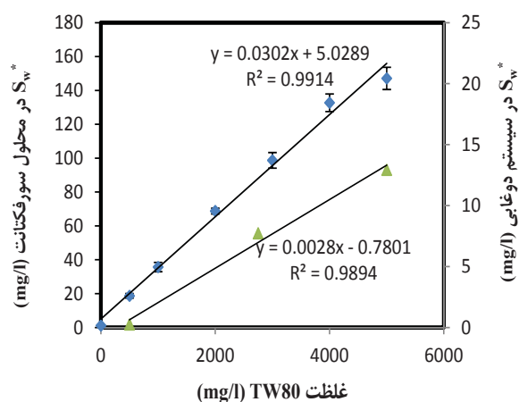
شکل ۱- ارتباط بین میزان حلالیت فنانترون و غلظت سورفاکتانت Tween 80 در محلول سورفاکتانت ▲ سیستم دوغابی، ۲۰ v/w: L/S
