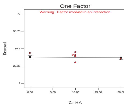
شکل ۶- تاثیر غلظت اسید هیومیک (HA) بر درصد حذف فنانترون، غلظت سورفاکتانت: ۲۰ v/w :L/S, ۲۷۵۰ mg/l, زمان شستشو: ۱۳ h
