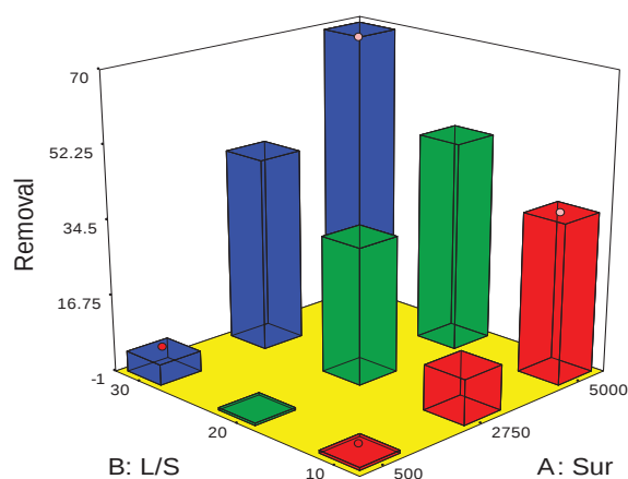
شکل ۳- تاثیر غلظت سورفاکتانتو نسبت L/S بر درصد حذف فنانترن، HA: ۱۰ mg/l، زمان شستشو: ۱۳ h
