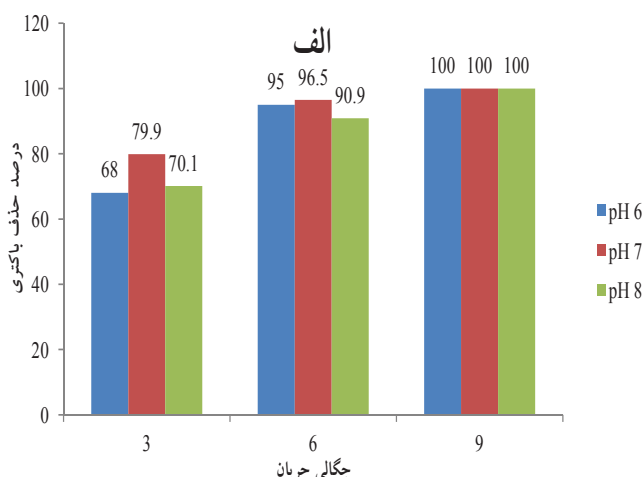
نمودار ۲ - درصد حذف باکتری پseudomonas آئروژینوزا در سیستم الکترولیز الف) 10^3 عدد در میلی لیتر، ب) 10^2 عدد در میلی لیتر در زمان الکترولیز 7/5 دقیقه، فاصله بین الکترودهای 1/5 سانتیمتر و چگالی جریان‌های مختلف
