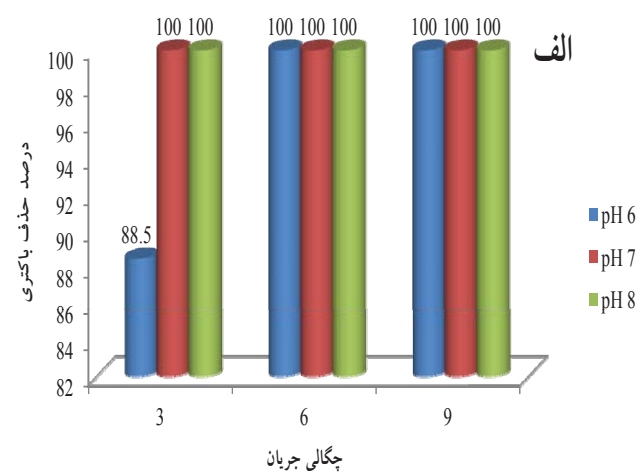
نمودار ۴ - درصد حذف باکتری پseudomonas آئروژینوزا در فوتوالکتروشیمیایی الف) 10^2 و ب) 10^3 عدد در میلی لیتر در زمان تابش 7/5 دقیقه، شدت تابش 600 میلی وات بر سانتی متر مربع و در pH و چگالی جریان‌های مختلف
