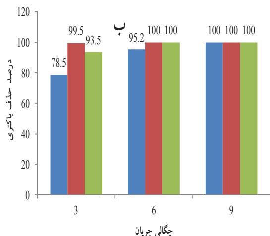
نمودار ۲ - درصد حذف باکتری پseudomonas آئروژینوزا در سیستم الکترولیز الف) 10^3 عدد در میلی لیتر، ب) 10^2 عدد در میلی لیتر در زمان الکترولیز 7/5 دقیقه، فاصله بین الکترودهای 1/5 سانتیمتر و چگالی جریان‌های مختلف
