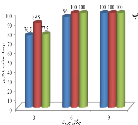
نمودار ۴ - درصد حذف باکتری پseudomonas آئروژینوزا در فوتوالکتروشیمیایی الف) 10^2 و ب) 10^3 عدد در میلی لیتر در زمان تابش 7/5 دقیقه، شدت تابش 600 میلی وات بر سانتی متر مربع و در pH و چگالی جریان‌های مختلف
