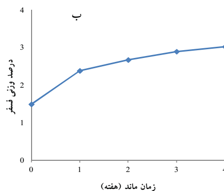
شکل ۳- تغییرات درصد وزنی فسفر در فرایند کمپوست، الف: نوده کمپوست هوازی ساکن، ب: توده هوازی توأم با اختلاط
