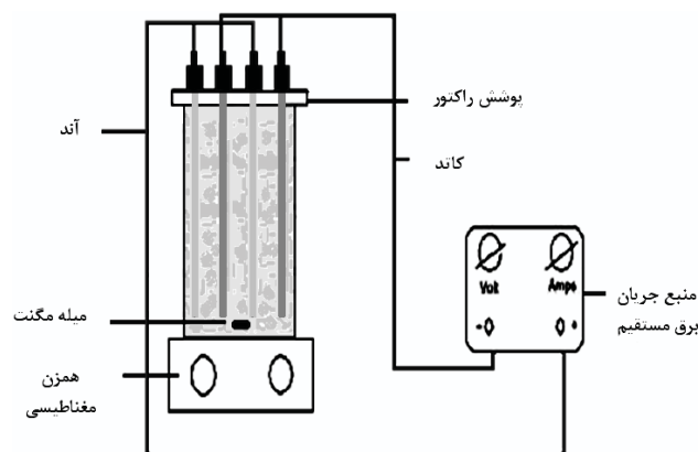
شکل ۱. شمای راکتور الکتروشیمیایی مورد استفاده جهت فرآیند انعقاد الکتریکی
